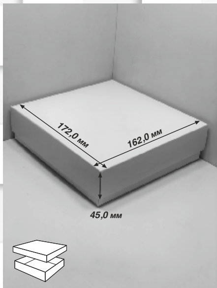
444 крышка и дно
