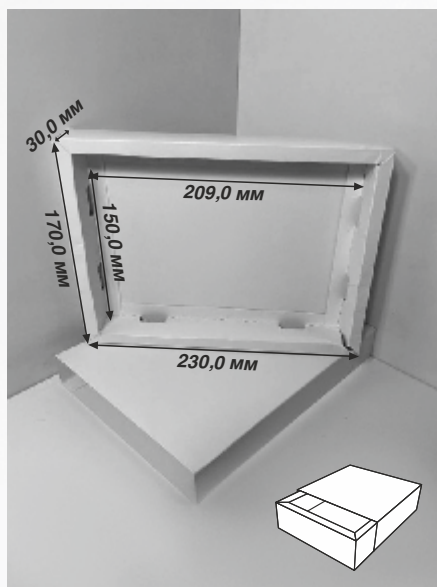
848 коробка и обечайка
