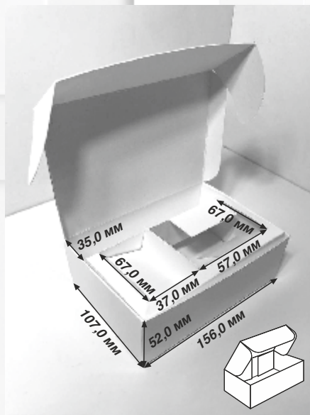
833 коробка и ложемент
