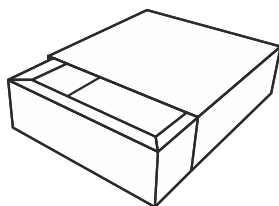
Коробка со съёмной крышкой в виде обечайки (пенал) Склейка обечайки Дно с двойным бортом
