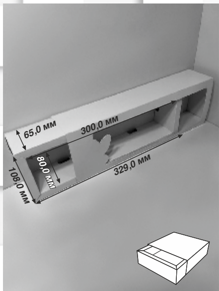
851 коробка и обечайка
