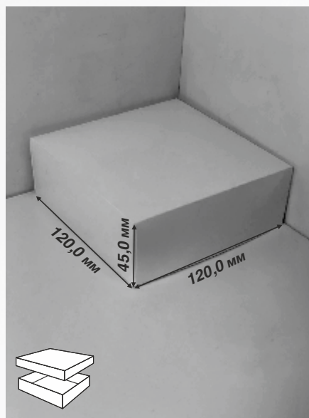
576 крышка и дно
