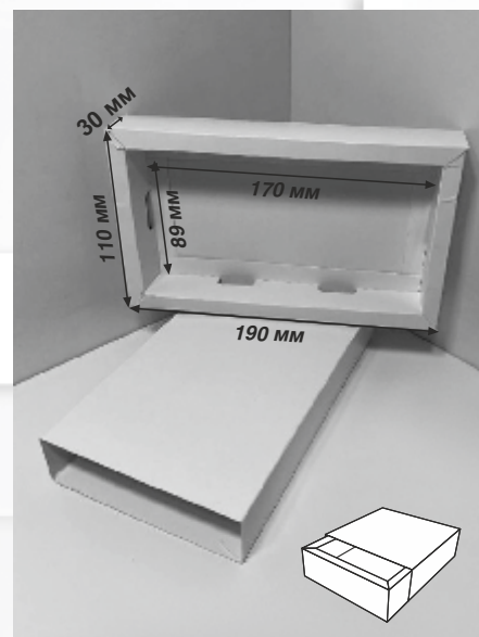
849 коробка и обечайка
